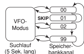
Ablauf im VFO-Suchlauf mit Speicherbanksuchlauf
