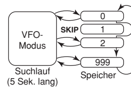
Ablauf im VFO-Suchlauf mit Speichersuchlauf
