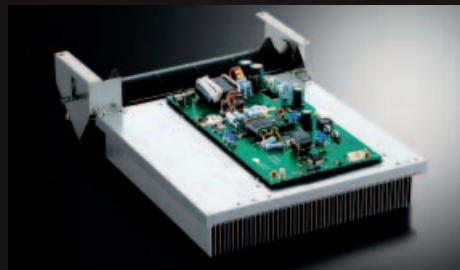
Endstufe und Kühlkörper
