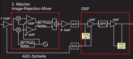
DIGI-SEL-Einheit
