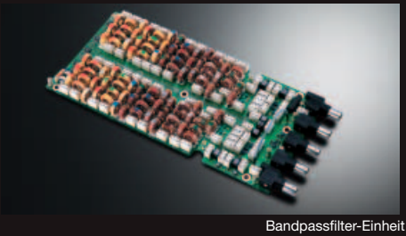
Bandpassfilter-Einheit
