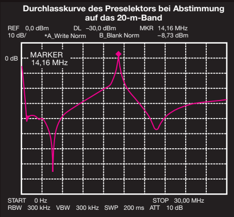
DIGI-SEL-Einheit
