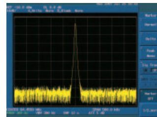
Durchlasskurve des 3-kHz-Filters (500 kHz Span)
