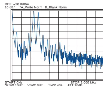
S9 +60 dBm-Eingangssignal
