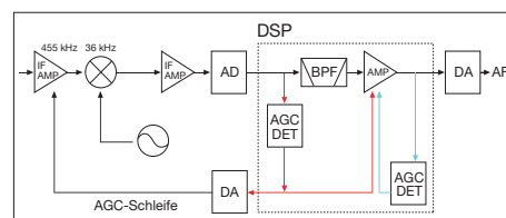
AGC-Prinzip
