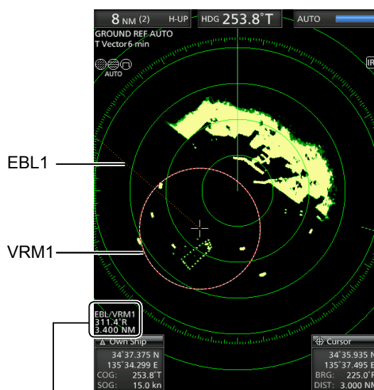
EBL1/VRM1 readout
