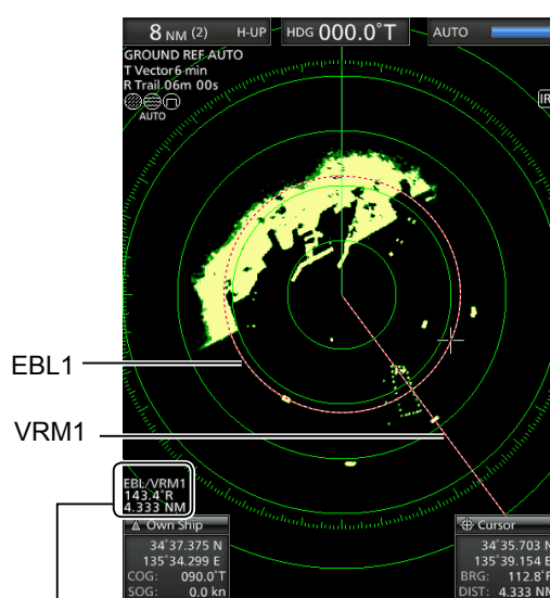
EBL/VRM1 readout
