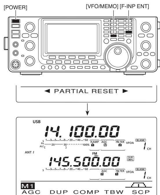
Anzeige der Initialfrequenzen von Haupt- und Subband
