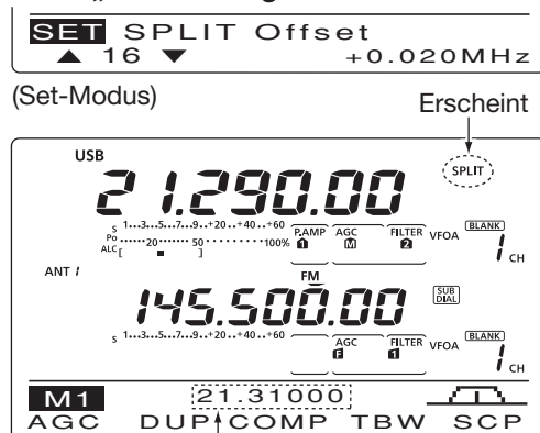
Anzeige der verschobenen Sendefrequenz (VFO B)
