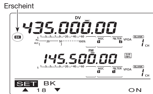
Break-in-Funktion ist eingeschaltet.
