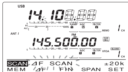
Beim \Delta F-Suchlauf
