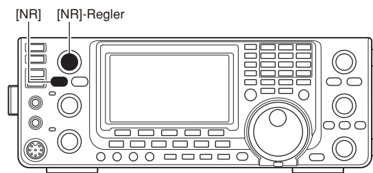
Rauschminderung aus Rauschminderung aktiviert
