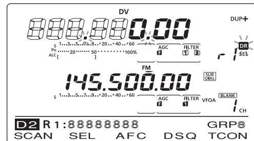
Display beim Einstiegs-Repeater-Suchlauf
