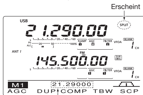
Anzeige der angeglichenen Sendefrequenz (VFO B)
