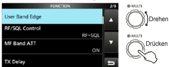
FUNCTION-Einstellbildschirm
